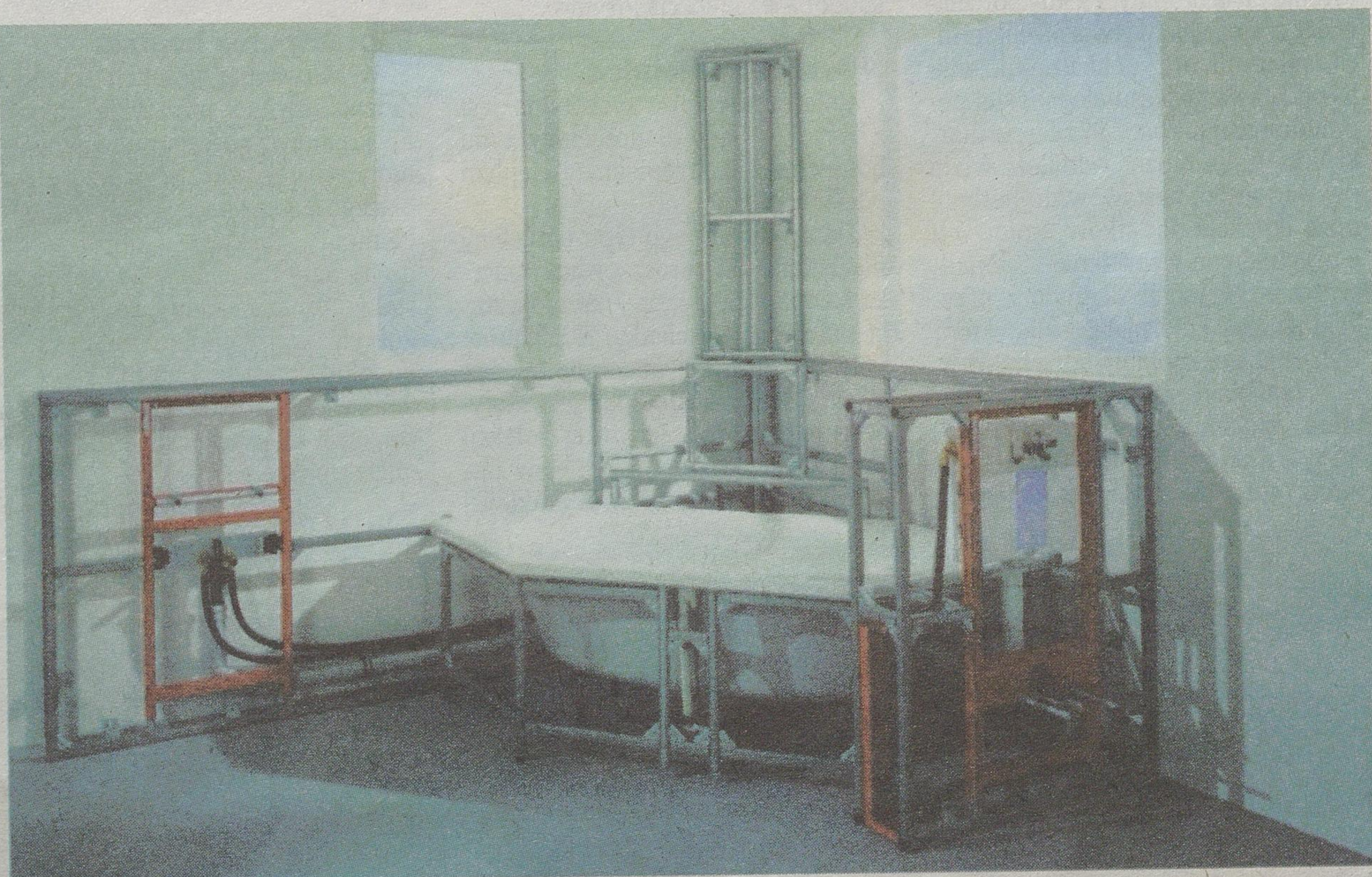
System TECEprofil jak na dłoni. Na metalowych profilach będzie można zabudować ścianki na przykład z płyty gipsowo-kartonowej. Czerwone elementy konstrukcji przeznaczone są do montażu takich elementów, jak umywalka czy muszla sedesowa.
