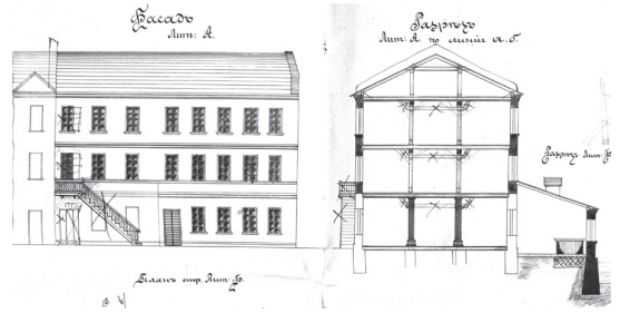
Projekt rozbudowy głównego gmachu produkcyjnego fabryki Henryka Litterera sporządzony w 1902 r. (źródło: Narodowe Archiwum Historyczne Białorusi w Grodnie, f. 8, op. 2, d. 1568, k. 14).
