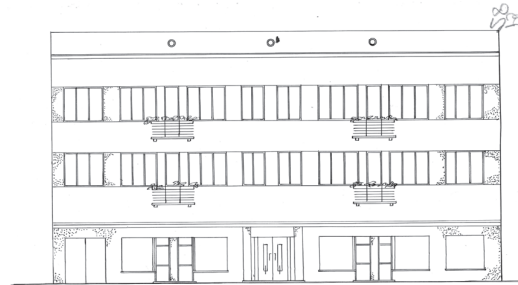
ELEVACJA FRONTOWA 1:100
