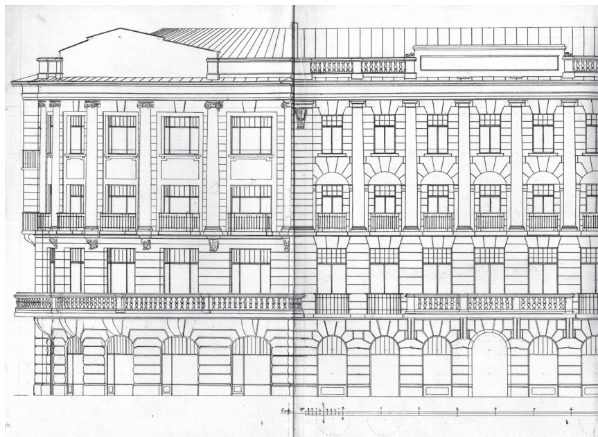
Fasada hotelu „Ritz” według inwentaryzacji z 1913 r. (źródło: Archiwum Państwowe w Białymstoku, Towarzystwo Kredytowe Miejskie Białostockie, sygn. 154, k. 4).
