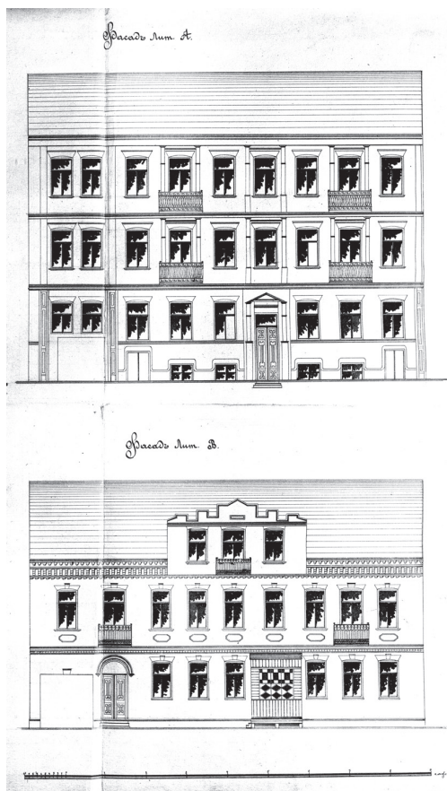
Rysunki elewacji frontowych obu kamien (frontowej i tylnej) Abrama Jossema z 1897 r. źródło: Litewskie Państwowe Archiwum Historyczne w Wilnie, f. 544, op. 1, d. 2436, k. 2).
