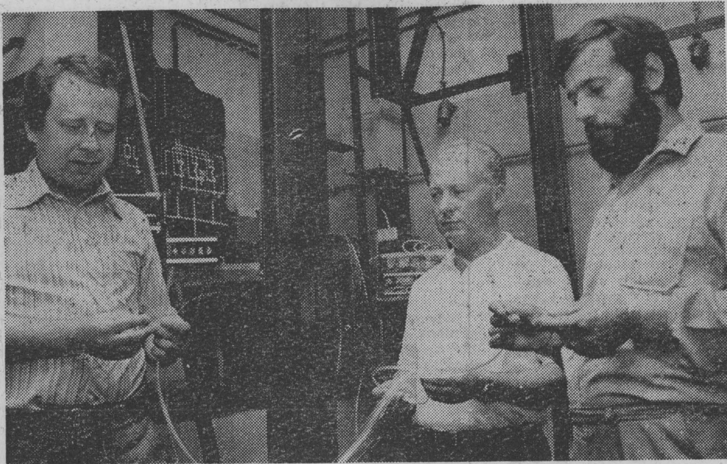
Jan Dorosz (z lewej), Wacław Leś i Jerzy Mazerski demonstrują zasadę działania światłowodowej wiązki.
