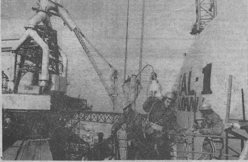
Monterzy z Mostostalu Kraków pracują przy budowie II wielkiego pieca.
