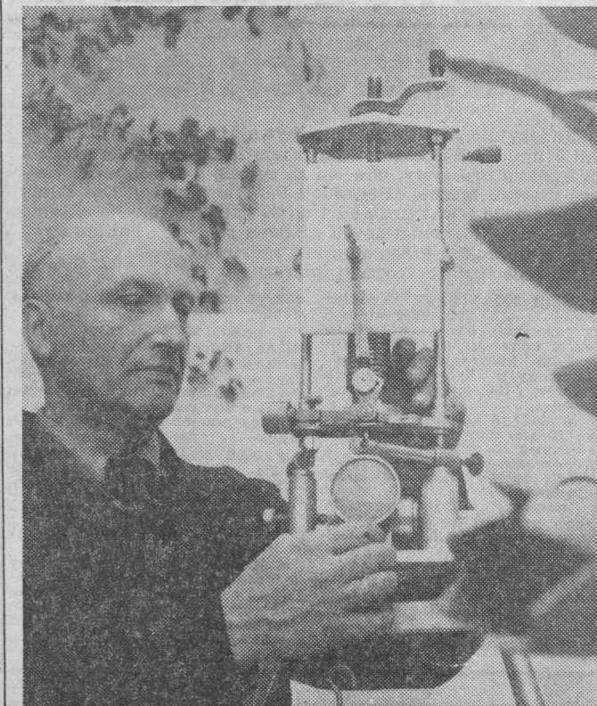
NA ZDJĘCIU: dr inż. Jacek Stróżecki przygotowuje do badań aparat do dwupłaszczyznowego ścinania gruntu przeznaczonych do badań laboratoryjnych.
