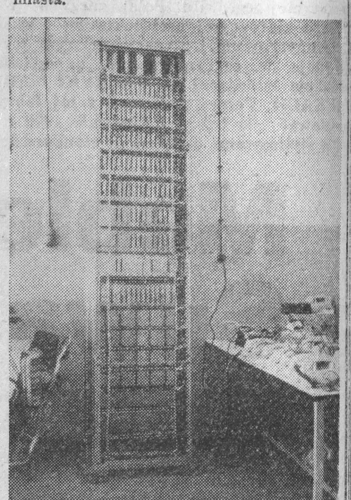
Stojak zakończeń kanałowych, który umożliwia podłączenie dodatkowych aparatów abonenckich.
