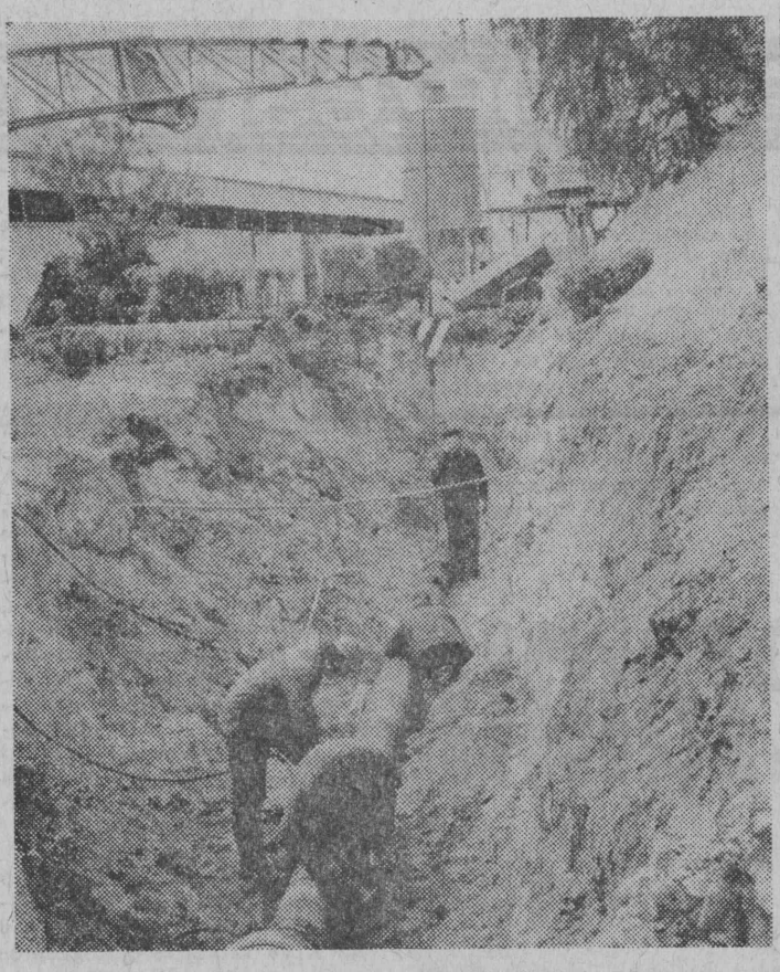
Brygada Mariana Tadysa podczas montażu jednego z trudniejszych odcinków gazowej magistrali — pod torami kolejowymi. Fot. Ryszard Łukowski
