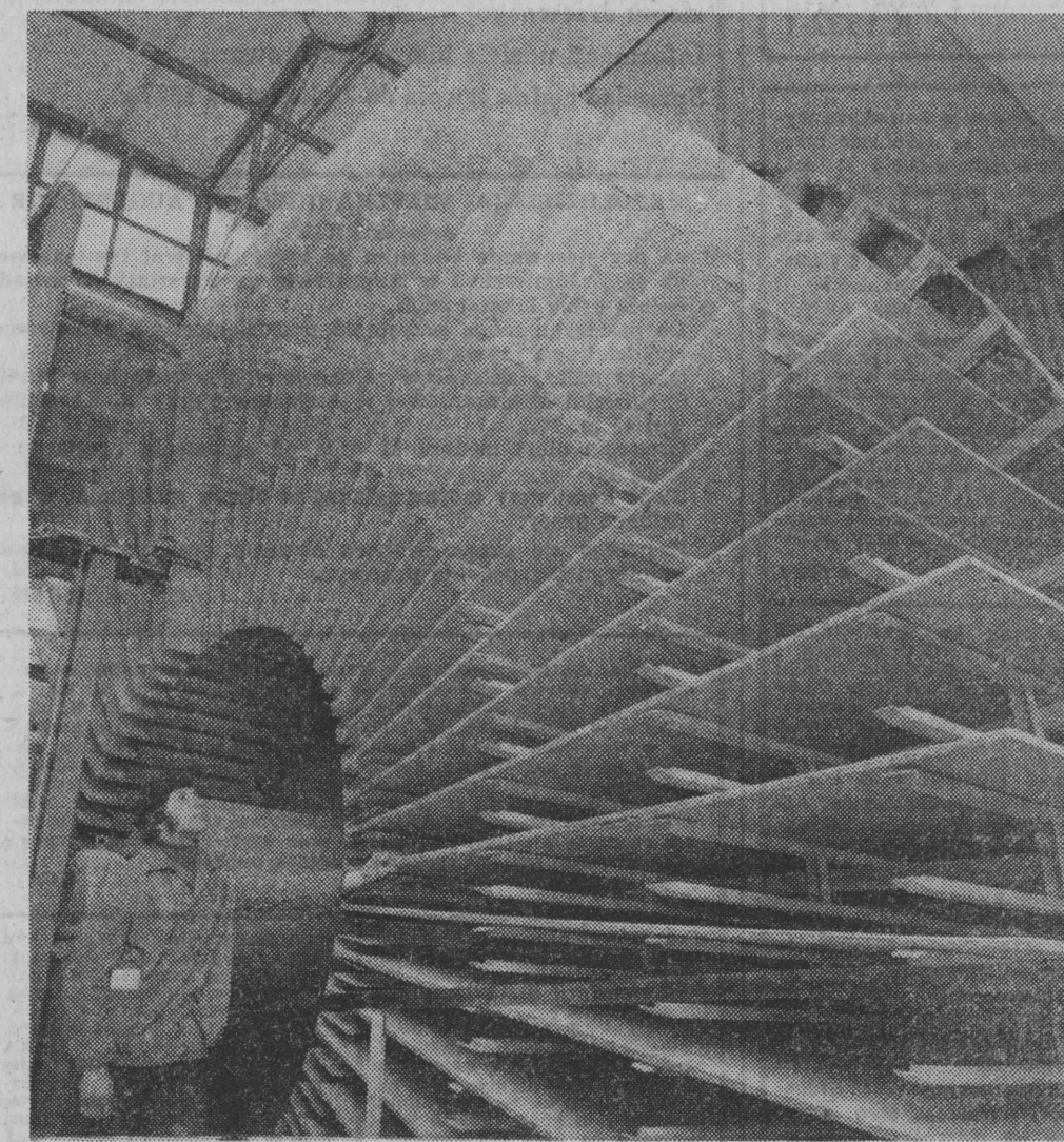
NA ZDJĘCIU: w grajewskiej wytwórni — z taśmy produkcyjnej płyty odbierane są przez tzw. młyn, a następnie trafiają do szlifowni, gdzie otrzymują wymaganą gładkość.
