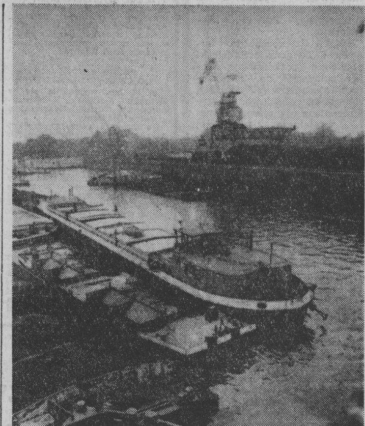
Jednym z największych portów na Odrze jest Koźle. W tym roku przeładowano tu już 900 tys. ton towarów, a w analogicznym okresie roku ubiegłego 500 tys. ton. NA ZDJĘCIU: praca w porcie. CAF — Okoński — tefefoto
