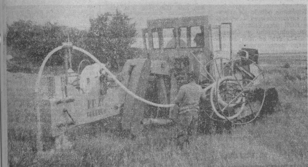
Tradycyjne konarki drenarskie wykonywały w ciągu dnia 500 metrów w rowku, w którym dopiero układano sie rzędy dreny ceramiczne. Na końcu rowek zasypywano... „Poldren KD-200” kładzie w tym samym czasie prawie 3 kilometry rur drenarskich z PCW, sam ko pie rowek i zasypuje go po całej szerokości. CAF — Łódź
