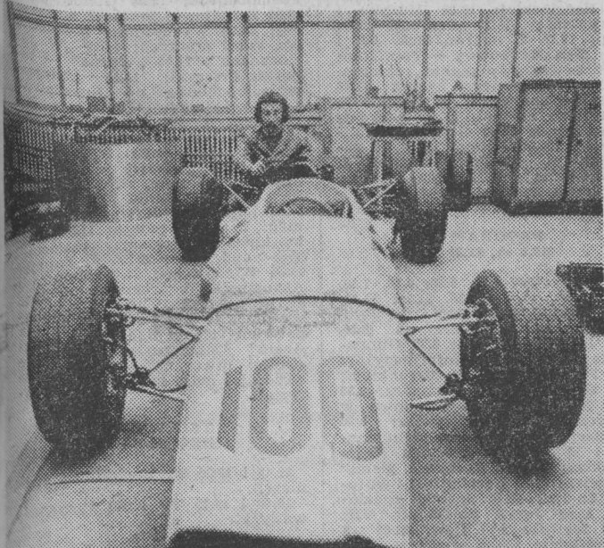
NA ZDJĘCIU: w Technikum Samochodowym im. Łojasza Kosutha w Budapeszcie uczniowie zbudowali prototyp samochodu wyścigowego wykorzystując w tym celu części i zespoły z radzieckiego samochodu „Żiguli”.
