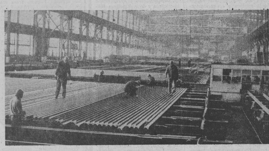
Huta „Kościszka” w Chorzowie — jeden z najstarszych tego typu obiektów w naszym budownictwie specjalizuje się w produkcji szyn kolejowych. Przeniesione one są na po-trzeby kraju i na eksport. M. in. do Brazylii. Wytop stali odbywa się w siedmiu piecach martenowskich. Wykończalnie walcownic opuszcza codziennie 1.200 ton wyrobów, większość to wspomina-ny już szyny, które ze względu na bezpieczeństwo ruchu kolejowego, przechodzą przed wysyłką dokładną i staranną kontrolę techniczną. NA ZDJĘCIU: kontrola techniczna szyn. CAF — Soko
