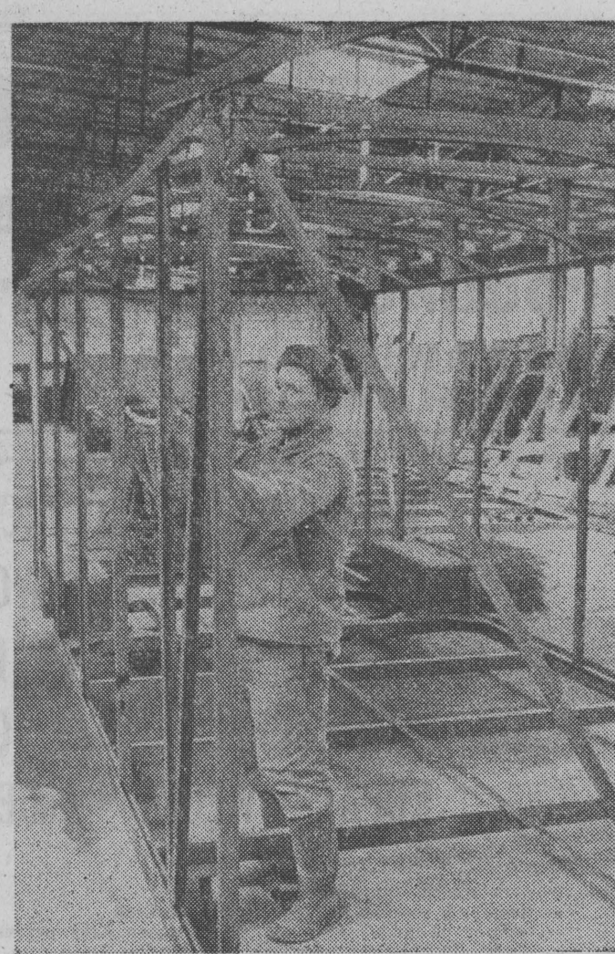
Hala spalalni. Właśnie tutaj przygotowują się konstrukcje pawilonów i barakowozów do dalszego wyposażania. NA ZDJĘCIU: — spawacz, Józef Pacetwicz, sprawdza prawidłowość wykonania szkieletu barakowozu.
