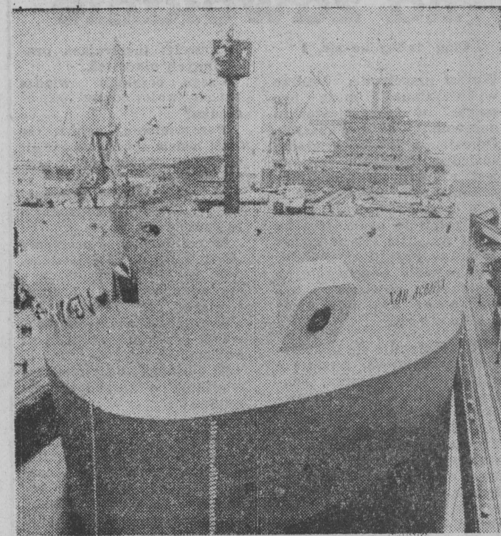
Pod koniec marca br. w Stoczni w Warnie zwodowano pierwszy bułgarski 100-tysięcznik noszący imię założyciela państwa — chana Asparucha. Tankowiec jest owocem współpracy polskich i bułgarskich stoczniowców. Jego projekt powstał w Stoczni Gdynskiej, a główny silnik napędowy o mocy 23 tys. KM pochodzi z zakładów „Cegleńskiego”. Bułgaria jest także eksporterem 25- i 38-tysięczników. CAF — BTA
