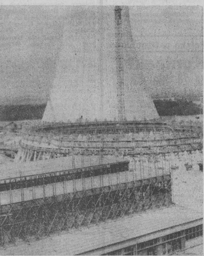
Na ostatnie dni czerwca br. planowany jest rozruch pierw-szego zespołu energetycznego o mocy 200 MW w obecnie bu-dowanej elektrowni Jaworzno III. Elektrownia ruszy do 1978 r. i osiągnie moc 1200 MW.
