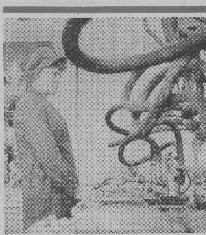
Łomżyńska Wytwórnia Zamknięć Koronowych jest jedną z dwu istniejących w kraju podległych Zjednoczeniu Piwowarskiemu. Rocznie wytwarza się 770 milionów sztuk popularnych kapsli. Plan realizowany jest z nadwyżką, w lutym uzyskano o dziesięć milionów sztuk więcej. Cały proces technologiczny jest zmechanizowany. W wyniku działań podjętych po II Plenum KC zmierzających do wykrycia rezerw, wytwórnia zaoferowała pięć milionów złotych (ten). NA ZDJĘCIU: w pracy wyróżnia się Agnieszka Wasik — operatorka gumiariek.
