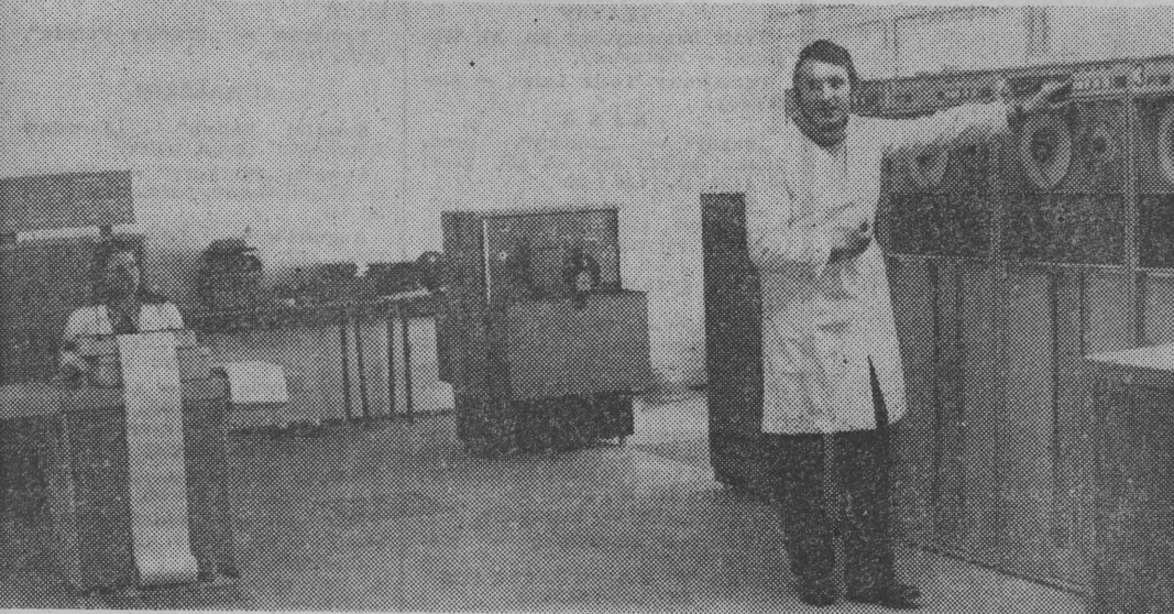
Fragment zestawu urządzeń „Odry” 13-05. Niewielka szafka w środku — to „mózg” maszyny.
