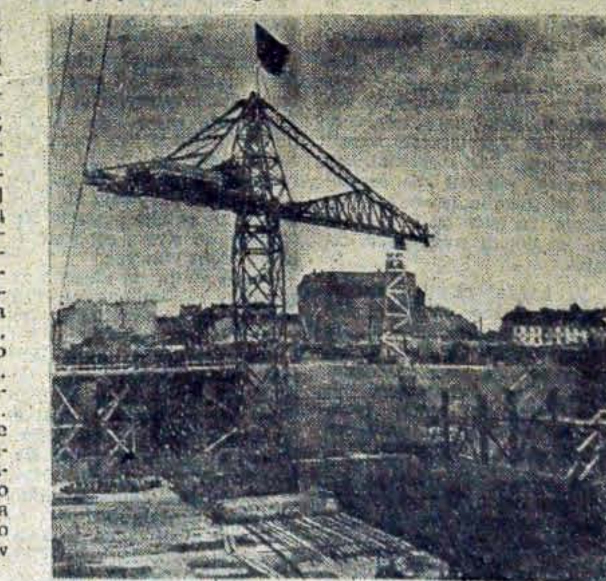
Fragment betonowania fundamentów pod Pałac Kultury i Nauki. Fot. — CAF
