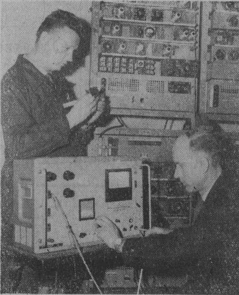
NA ZDJĘCIU: mgr inż. Kazimierz Maciejewicz i st. technik Aleksander Szczepiński przy pracy nad przebudową urządzeń telefonii nośnej.
