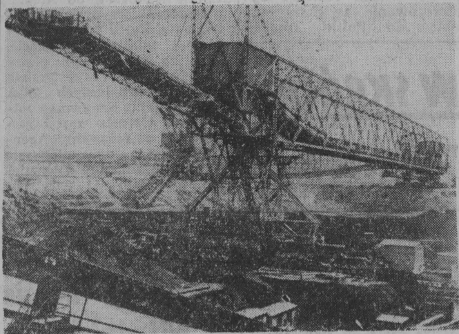
Ta wielka koparka krocząca została wykonana przez Fabrykę Ciężkich Maszyn w Lauhammer (NRD). Koparka-gigant pracuje w odkrywkowej kopalni węgla brunatnego „Schwarze Pumpe”.
