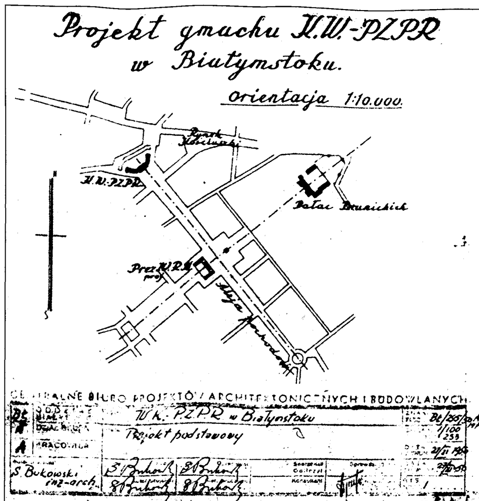
Plan sytuacyjny gmachu KW PZPR w Białymstoku w skali 1 : 10000 wykonany przez Stanisława Bukowskiego. (Oryginał znajduje się w dziale inwestycji, remontów i konserwacji Uniwersytetu w Białymstoku)
