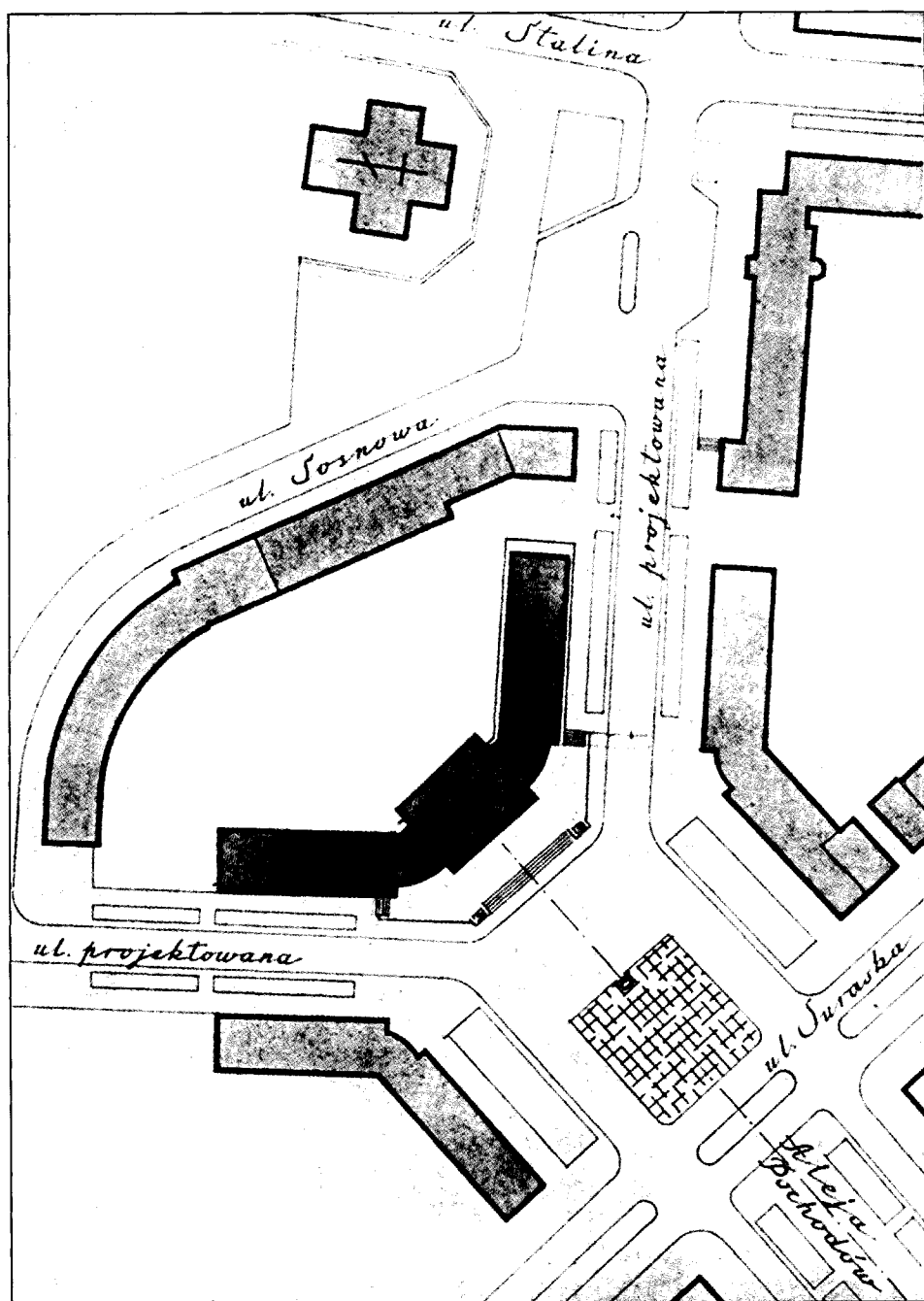
Plan sytuacyjny budynku KW PZPR w skali 1 : 1000 wykonany przez Stanisława Bukowskiego. (Oryginał znajduje się w dziale inwestycji, remontów i konserwacji Uniwersytetu w Białymstoku)
