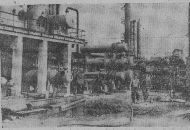
NA ZDJĘCIU: fragment instalacji do uwodorniania wyższych frakcji (reforming) w Zakładach Petrochemicznych w Płocku. CAF — fot. Rosiak
