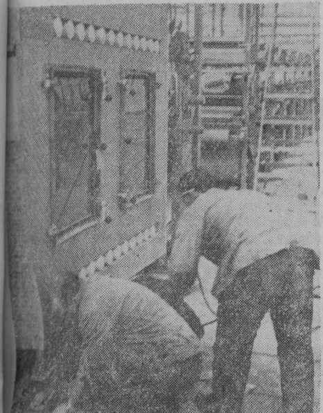
Andrychowskie Zakłady Przemysłu Bawełnianego w Andrychowie 47 proc. produkcji przeznaczają na bezpośredni eksport w większości do krajów strefy dolarowej. Obecnie buduje się nową wykończalnię. NA ZDJĘCIU: montaż urządzeń ciągłych do barwienia tkanin w nowej wykończalni. CAF — fot. Olszewski
