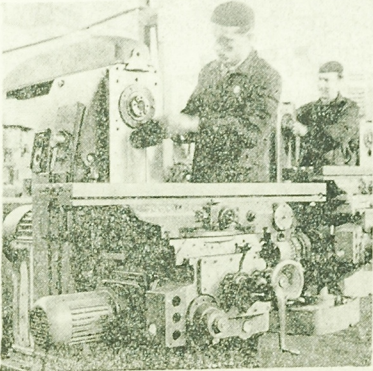
Jazelska Fabryka Obrabiarek produkuje kilka wersji frezarek — posuwowe, poziome i unieruchamione. Ostatnio zainstalowano 3 prototypy, które wejdą do produkcji w bieżącym roku, a opracowane zostały przez pracowników CHKO. Ponad 20 proc. produkcji zakładu przeznaczony jest na eksport do 75 krajów na wszystkich kontynentach (m. in. do Włoch, USA, Szwecji i NRD). CAP — Sławyżny
