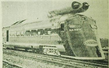
Amerkańskie towarzystwo kolejowe New York Central przeprowadza próby nowego typu lokomotywy o napędzie odrzutowym (na zdjęciu). Podczas próby na linii Butler (stan Indiana) lokomotywa (stan Ohio) osiągnęła szybkość 275 km/godz. CAP - AFP
