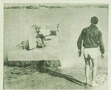
John Newman z Claremont (Australia) z zawodu inżynier-elektryk, konstruuje podziemne własnego projektu, 4-cylindrowy silnik samochodowy unosi pojazd nad ziemią, a motocyklowy silnik o pojemności 150 cm pozwala osiągnąć szybkość do ponad 70 km/godz.
