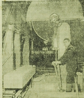
Wacław Budziński obsługiwał nowoczesny trakt, w którym przeciera się drewno liściaste.
