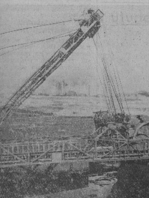
NA ZDJĘCIU: koparki kroczące przy pracy na odkrywe „Turów I”, w głębi widać po drugiej stronie granicy dymiące komin elektrowni w Hirschfelde. CAF - fot. Wołoszczuk
