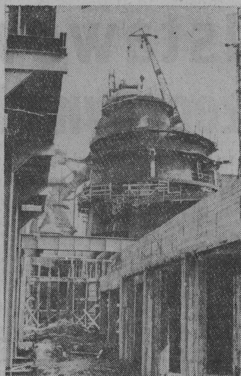
W hucie im. Lenina główne prace przy dalszej jej rozbudowie koncentrują się przy IV wielkim piecu. NA ZDJĘCIU: budowa IV wielkiego pieca. CAF — fot. Dąbrowiecki
