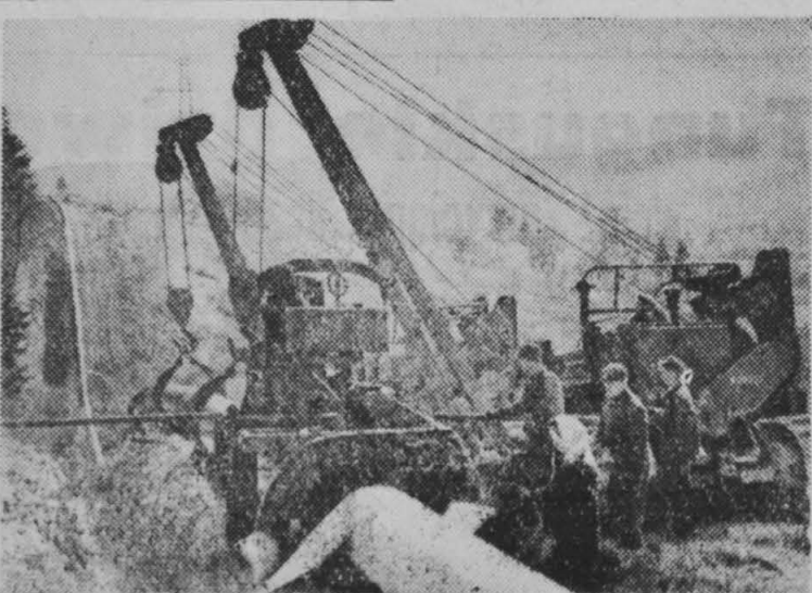
NA ZDJĘCIU: robotnicy brygady Z. Leszegi okręcają rurociąg izolacją i przy pomocy specjalnych dźwignów — ukladają go w ziemi.
