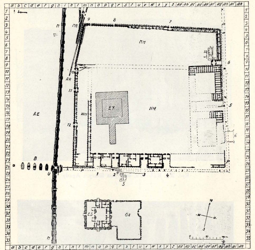
Ryc. 279. Babilion, Etemenanki i Esagila (plan; por. ryc. 269, 89, 90—96, 172, 174, 296)
