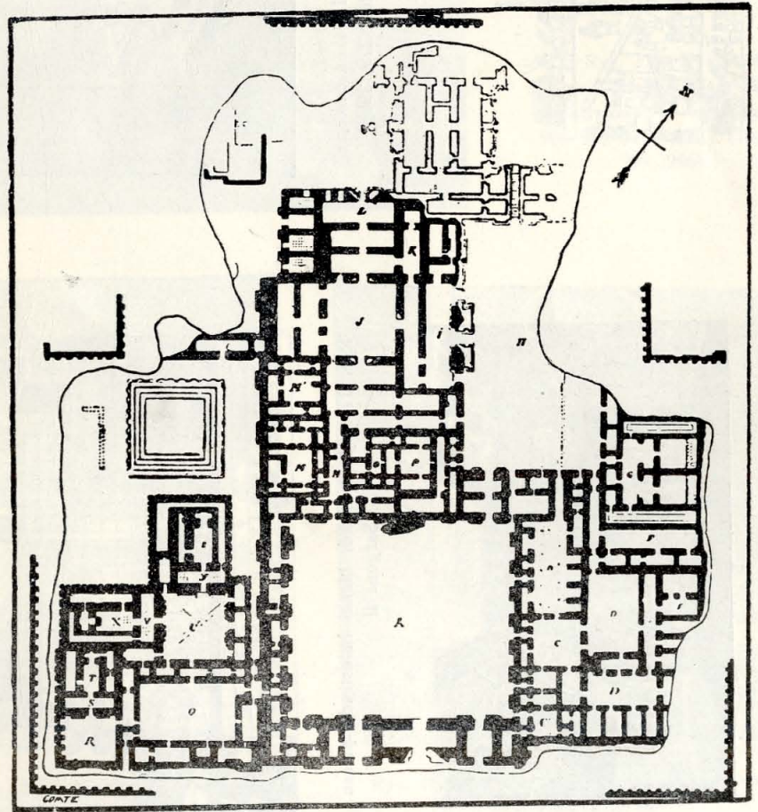
Ryc. 173. Ҳorsâbâd, plan pałacu Sargona II i 3 świątyń (por. ryc. 86)
