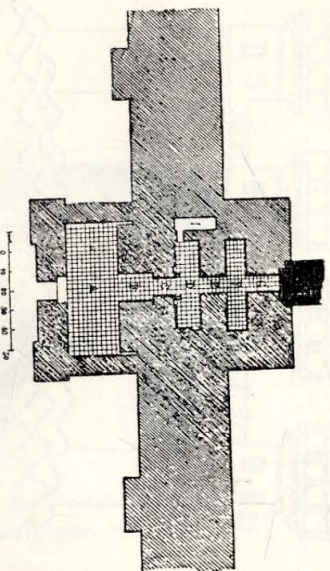
Ryc. 200. Horsaġād, brama miasta obwarowanego (przecięcie poziome; — por. ryc. 157, 170, 199)
