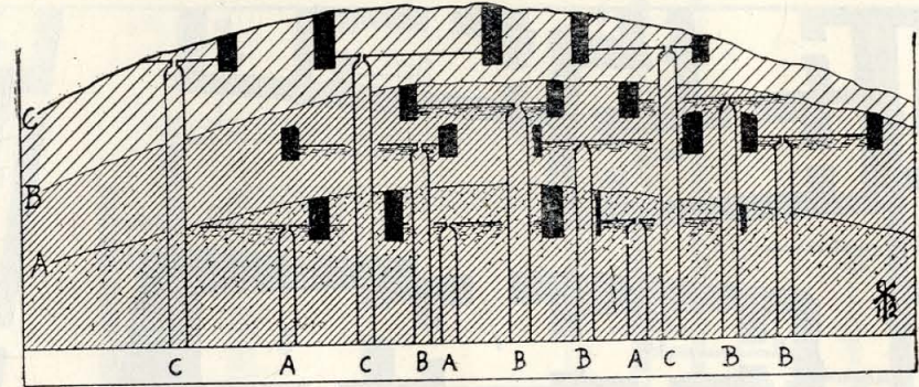
Ryc. 283. Babilon, schematyczny przekrój studzien we warstwach ruin
