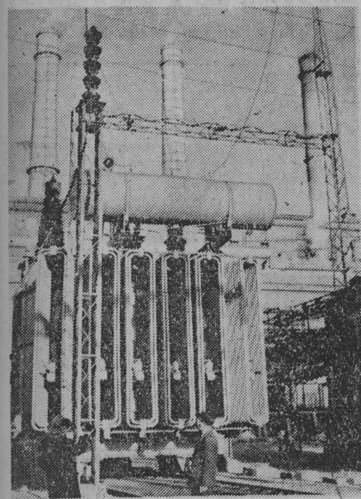
W największej naszej siłowni Jaworzno II wybudowanej i włączonej do eksploatacji w Planie 6-letnim, w dniu 5 bm. zakończono montaż i rozpoczęto ruch ostatniego turbozespołu. Elektrownia Jaworzno II została zbudowana w oparciu o dokumentację radziecką. Związek Radziecki dostarczył również podstawowych maszyn i urządzeń. NA ZDJĘCIU: fragment rozdziału siłowni Jaworzno II. CAF toł. Tymiński
