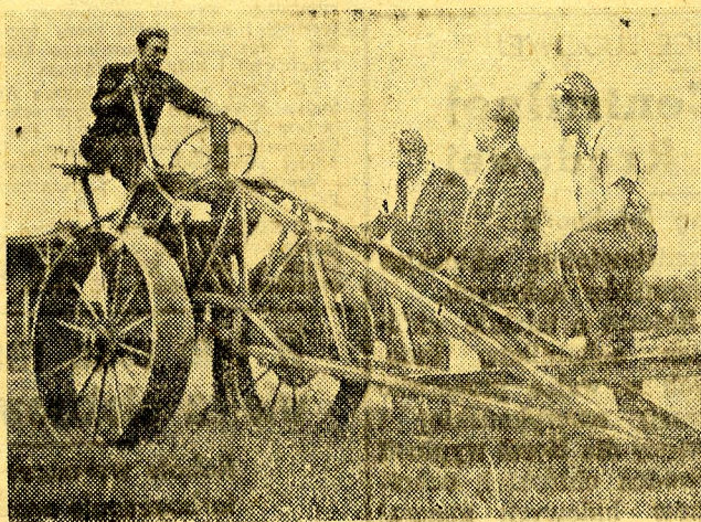
Kwapiszewski (drugi od prawej) udziela traktorzystom znanonowi Sztorcowi wskazówek dotyczących obsługi i działania pluga własnej konstrukcji do kreciego drenowania.
