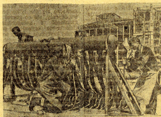
Na zdjęciu: Kazimierz Osiecki (wykonujący 240 proc. nowej normy) i Jan Owczarczyk (przekracza podjęte w czy- nie lipcowym zobowiązanie wykonywania 250 proc. normy) z brygady Miśkiewicza, przy spawaniu rur ekranu kotła si- lowni. W głębi siłownia w budowie.
