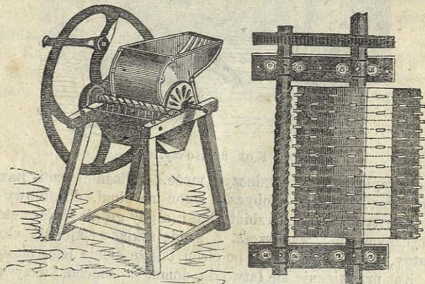
Szarpacz czyli rozdrabiacz Bentall'a.
