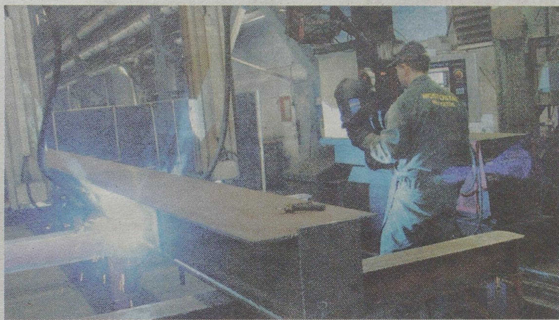
Portal spawalniczy na pewno usprawni pracę, ale nie zabierze jej spawaczom. Człowiek musi nadzorować pracę maszyny.
