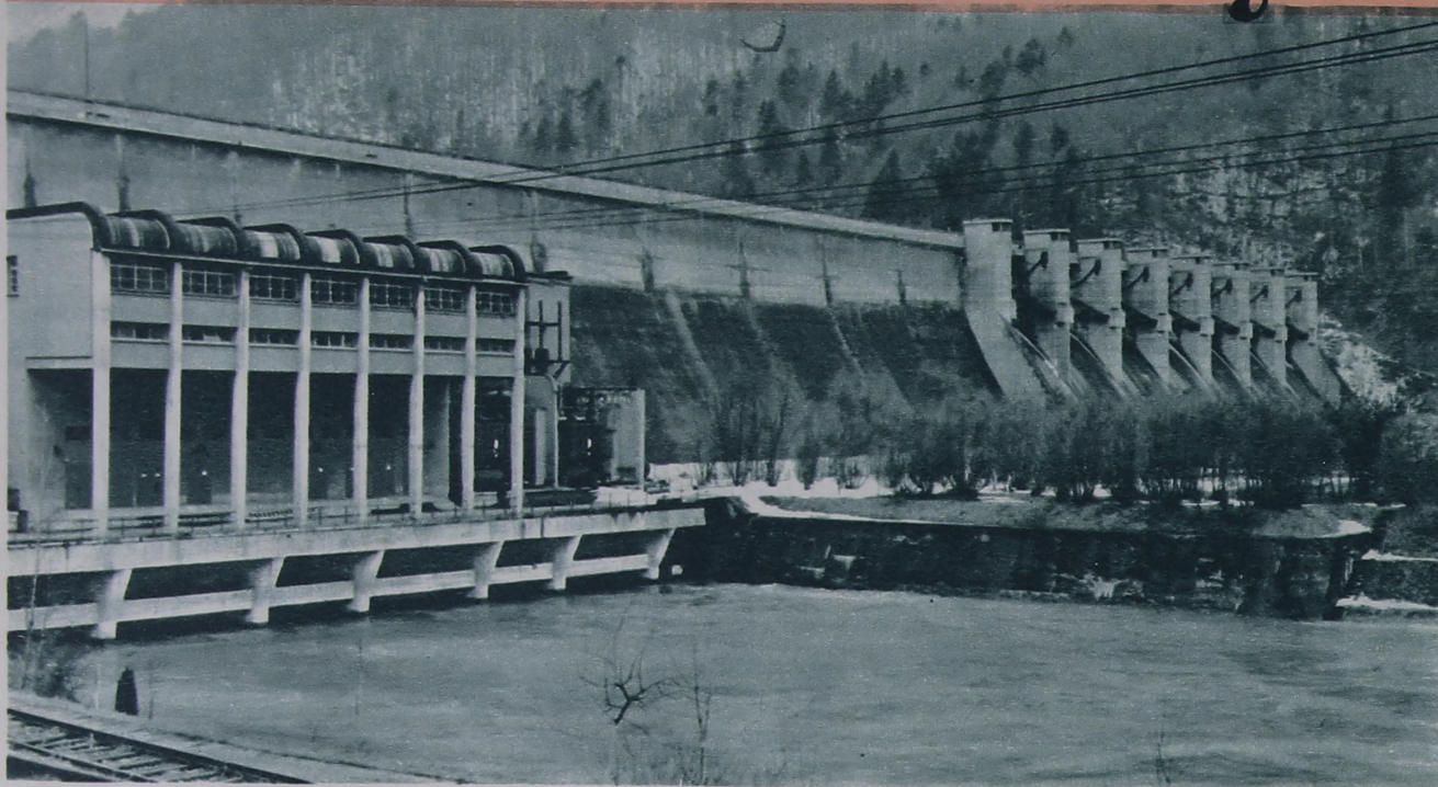
U góry: Zapora i elektrownia wodna na Dunajcu w Rożnowie Po lewej: Zapora i elektrownia wodna w Solinie
