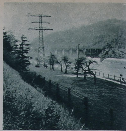
U góry: Zapora wodna w Porąbce U dołu: Włocławek. Teren budowy
