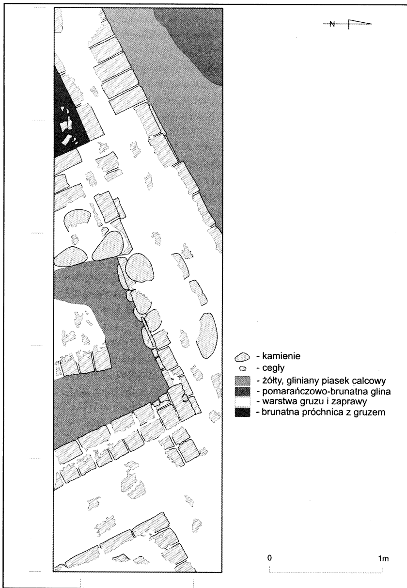
Ryc. 12 – Czerłona. Wykop 2, rzut.
