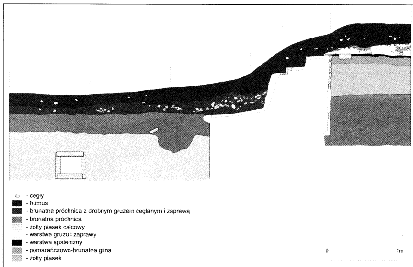
Ryc. 8 – Czerlona. Wykop 1, profil S.
