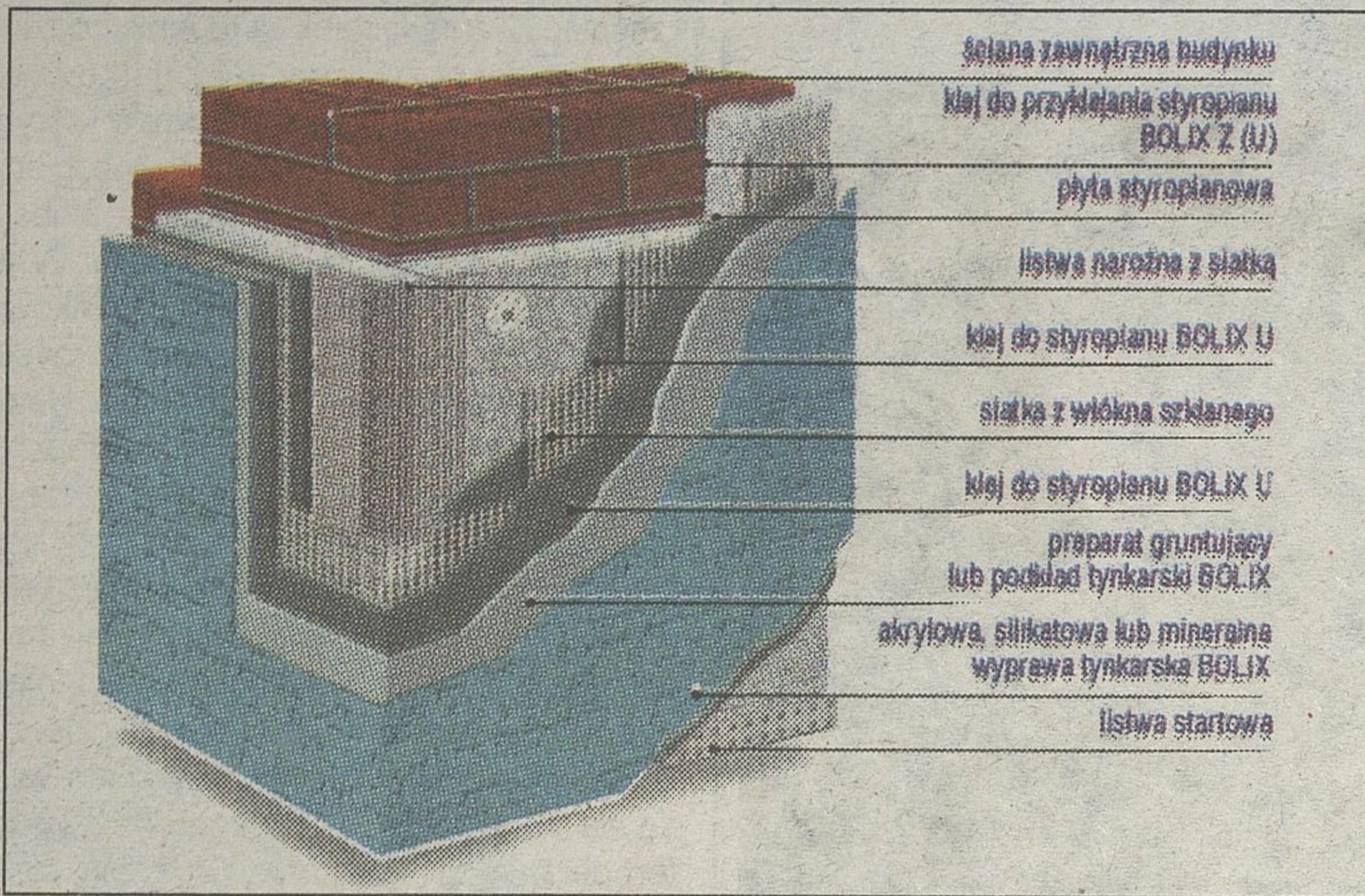
Przekrój systemu dociepleniowego Bolix
