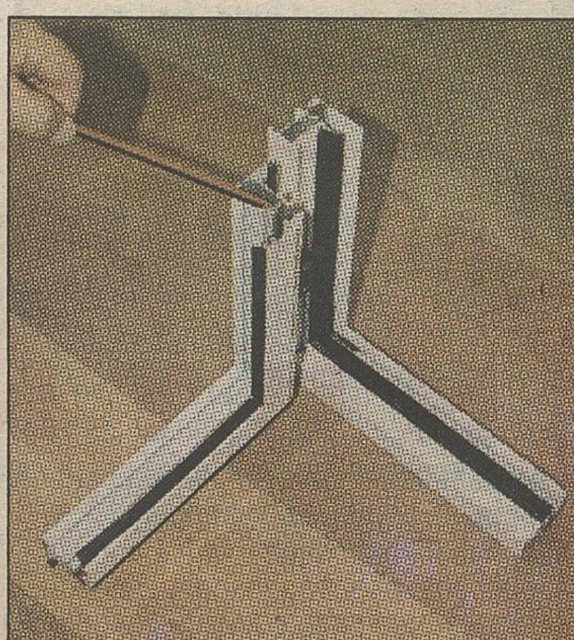
Aluminiowy profil belgijskiej firmy Reynaers z wkładką termiczną
