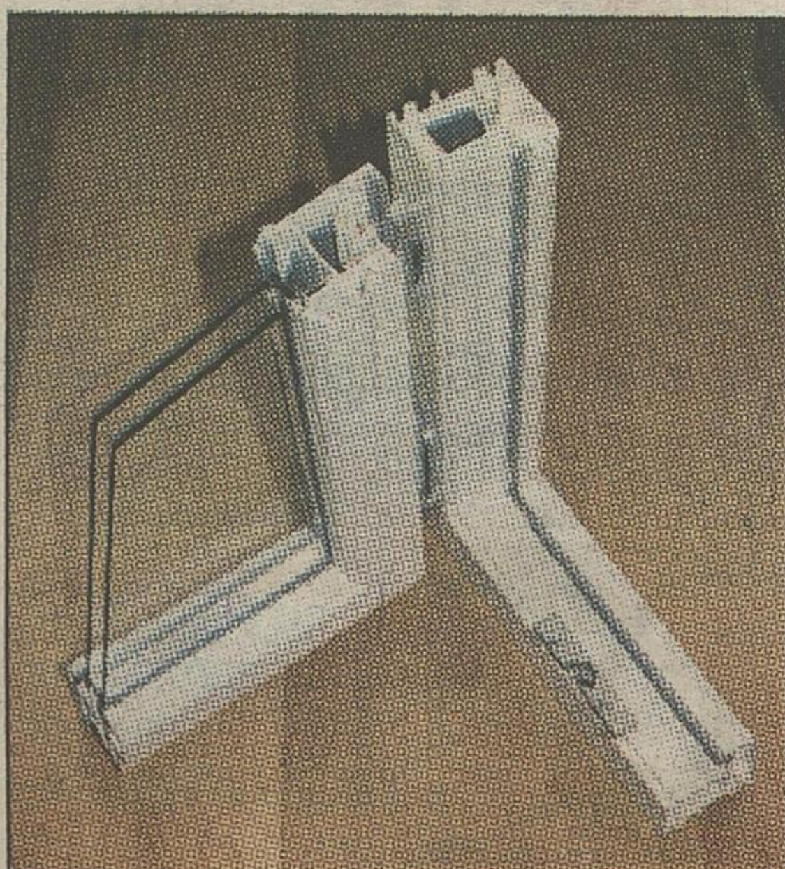
Przekrój trzykomorowego profilu niemieckiej firmy KBE
