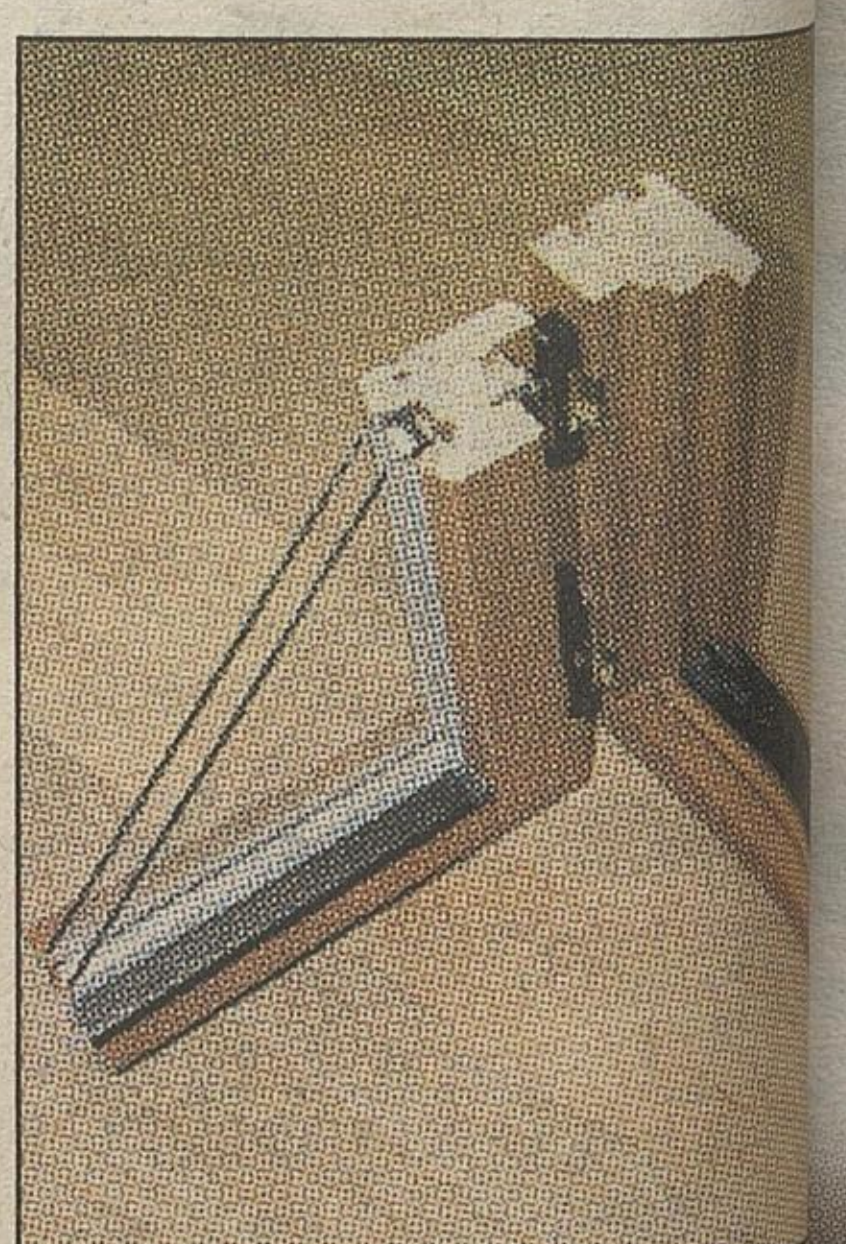
Przekrój okna z drewna sklejonego warstwowo
