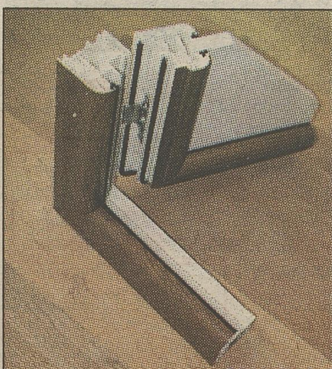
Sześciokomorowy profil niemieckiej marki Aluplast 6000
