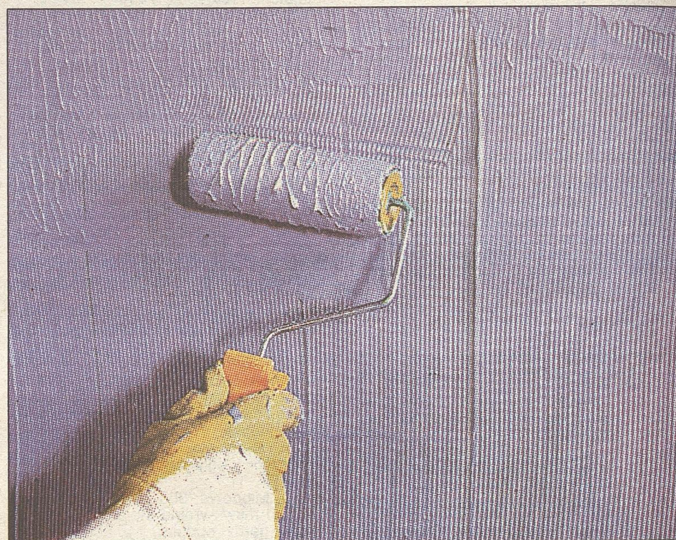
Rozprowadzanie izolacji wodoszczelnej
