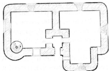
Średni schron bojowy do ognia dwuboczny z kopułą pancerną dla jednego ckm. Obiekt jednokondygnacyjny. Rys. E. Stefanowicz, 2003
