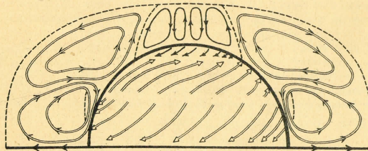
Ryc. 34. Ogólny system krążenia powietrza na powierzchni ziemi na północ od równika. Zauważ a) kierunki wiatrów na powierzchni ziemi, b) ruch powietrza ponad ziemię. Linje kropkowane w pobliżu bieguna oznaczają granicę frontu polarnego.
