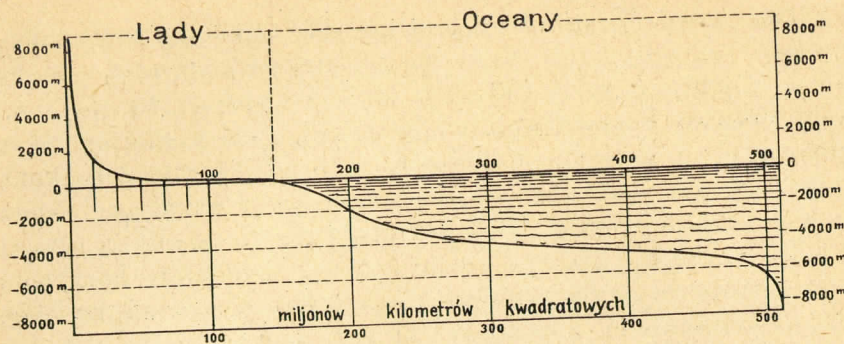
Ryc. 13. Krzywa hipsograficzna.
