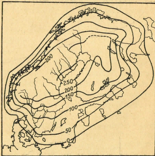
Ryc. 19. Podnoszenie się Skandynawji po epoce lodowej. Cyfry oznaczają metry n. p. m.
