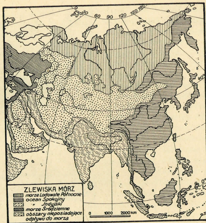
Ryc. 78. Zlewiska mórz i obszar bezodpływowy.
