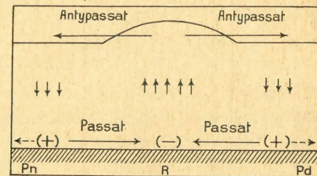
Ryc. 33. Krążenie powietrza na ziemi w pobliżu równika. Znak (+) oznacza wysokie ciśnienie, znak (—) niskie ciśnienie, strzałka kierunek ruchu powietrza.
