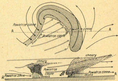
Ryc. 31. Na górnej rycinie widzimy (w rzucie poziomym), jak powietrze ciepłe na powierzchni ziemi napływa do środka cyklonu od południowego zachodu. Dolna rycina daje przekrój: A A' przez cyklon i wyjaśnia powstanie deszczu.
