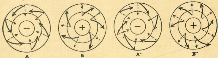
Ryc. 32. Ruch cyklonalny (—) i antycyklonalny (+) wiatru na półkuli północnej (AB) i na półkuli południowej (A'B'). Strzałka przerywana oznacza kierunek normalny, strzałka pełna kierunek odchylony.
