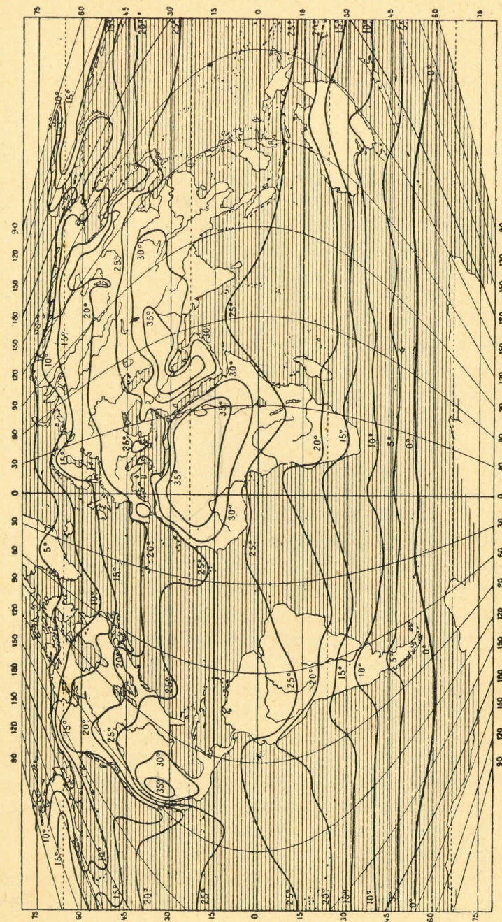
Ryc. 29. Izotermy lipca na kuli ziemskiej.
