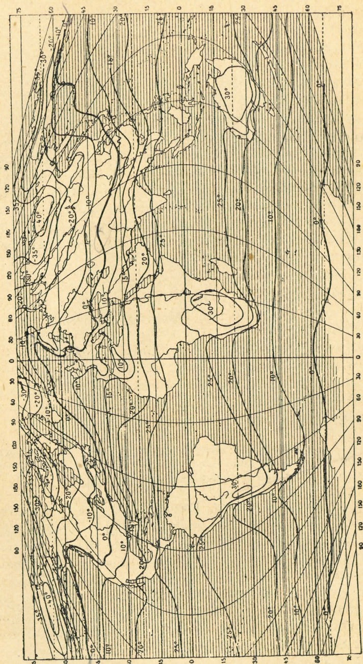
Ryc. 28. Izotermy stycznia na kuli ziemskiej.
