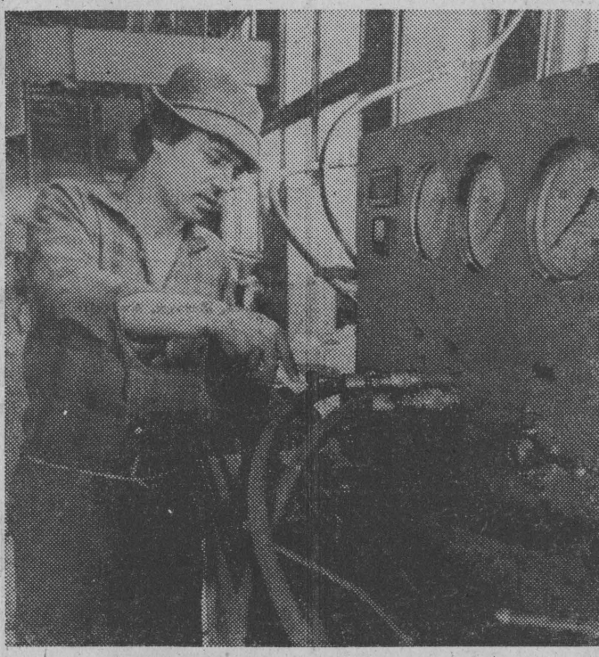
Instalacja hydrauliczna do ładowacza, którą sprawdził Waldemar Antoniuk, czeka na podnośnik z Lubania Śląskiego. Dotychczas było, że okres ten wydłużał się dość znacznie.
