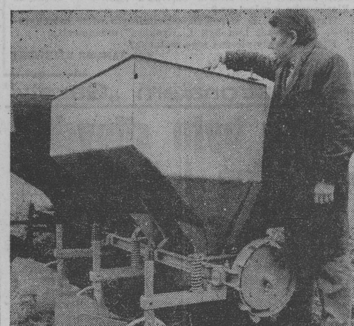
Inż. Witold Bakun prezentuje prototyp sadzarki dwurzędowej do ziemniaków.
