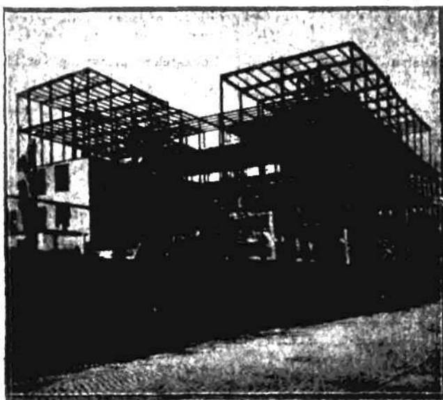
Budowa pierwszego w Warszawie domu murywanego o całkowicie żelaznej konstrukcji, prowadzona przy zbiegu ulic Poznańskiej i Nowogrodzkiej, postępuje szybko naprzód. W gmachu tym ma być pomieszczenia główna centrala telefonów międzymiastowych.
