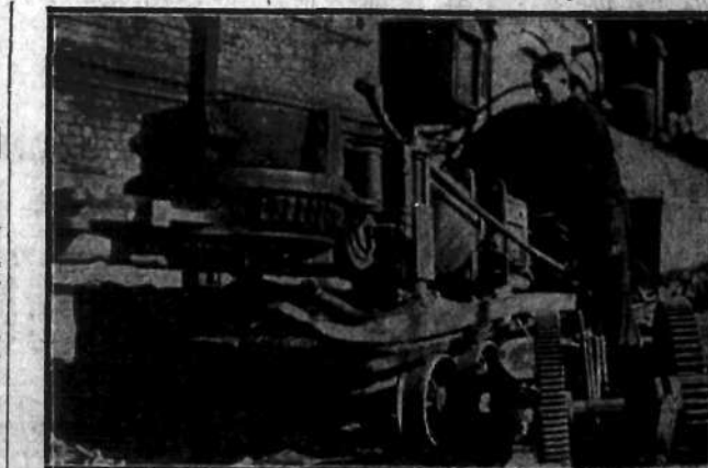
Maszynierza kopalniana, która spowodowała straszną katastrofę w szybu „Kurt” w Hausdorf na Śląsku Opolskim. Jest to t. zw. „wagon Schramma”, bo iacy otwory w pokładach węgla przy pomocy elektrycznego świdra. Maszyn tych w kopalniach obecnie używać nie wolno.
