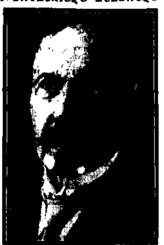
KAROL RICHERT , wielki uczonec francuski, laureat Nobla, obchodził ostatnio 75 rocznicę urodzin. Do najznakomitszych dzieł twórcy teorii seratacji należały: „Trucizna inteligencji”, „Fizjologia mięśni i nerwów”, „Słownik fizjologiczny” i inne.
