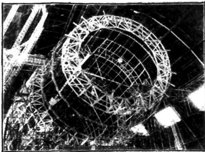
Szkielet olbrzymiego sterowca, który ma być wykończony w 1933 r., montowany z pośpiechem w zakładach lotniczych w Akron w stanie Ohio w Ameryce Północnej.
