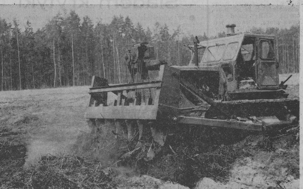
Karczowniki można zastosować na dużych terenach przygotowywanych pod szkółki leśne.
