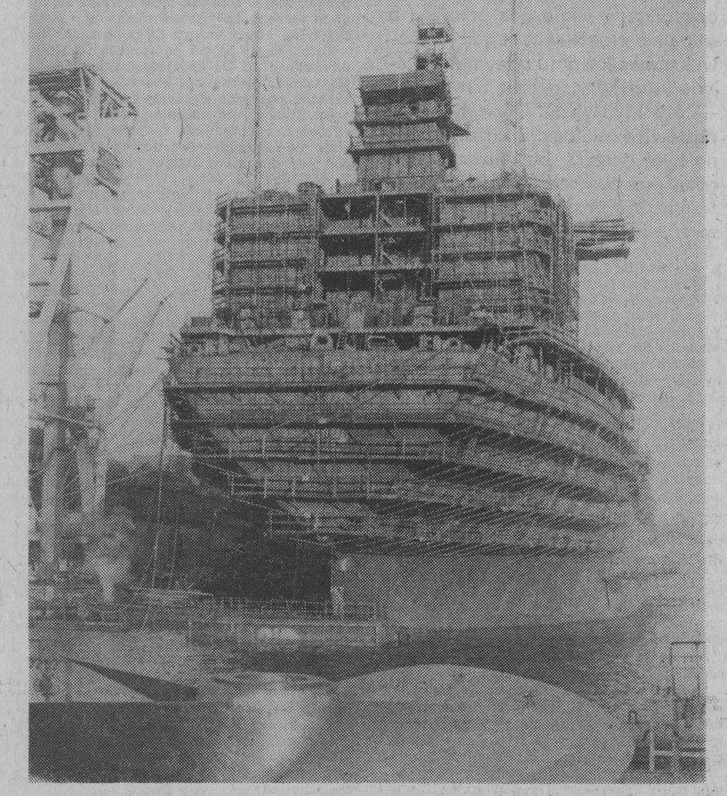
Kolejny statek-gazowiec w basenie wyposażeniowym Stoczni im. Komuny Paryskiej w Gdyni. Budowa tych niezwykle skomplikowanych jednostek stała się jedną ze specjalności polskiego przemysłu okrętowego.
